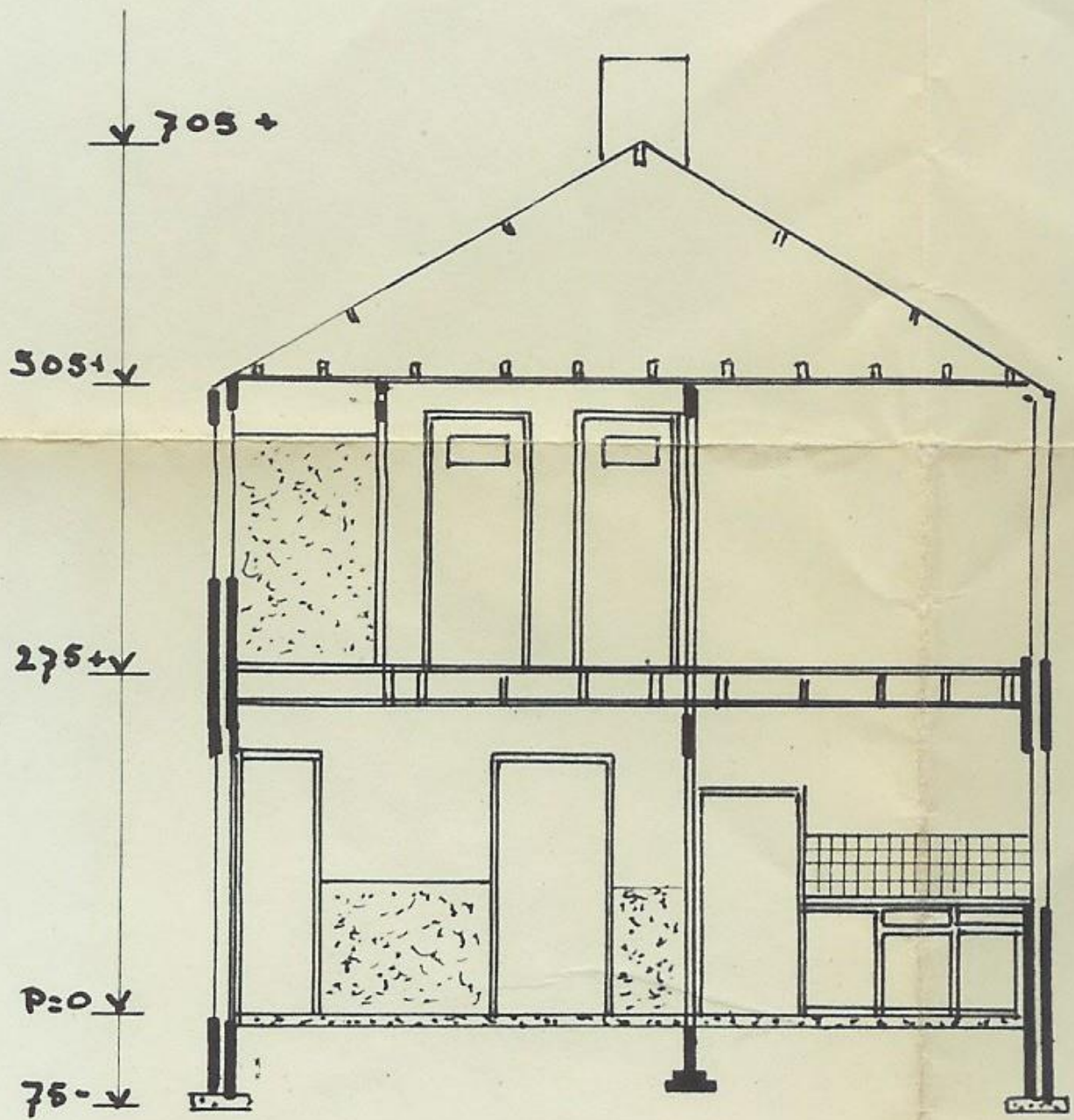
DOORSNEDE A-A
